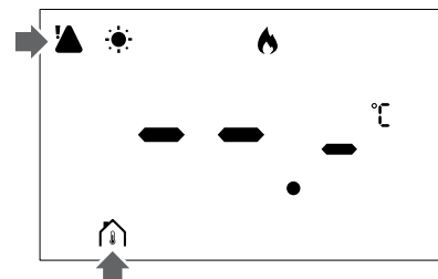
Joonis 2. Näide RT juhtimisrežiimiga küttesüsteemist, mis töötab ilma nõudluseta mugavusrežiimis
